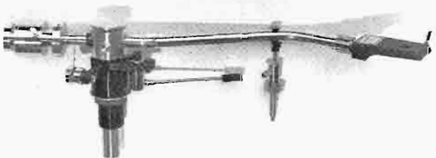
Russco RA-12 Tone Arm
