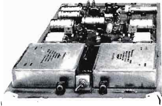
786V-1 Stereo Generator
